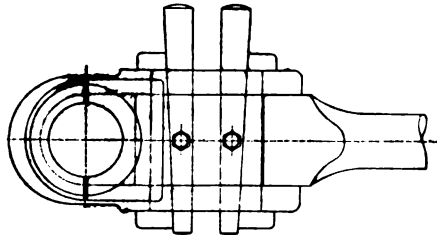
Č. 1712. Hlava ojnicní.
